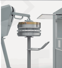
Sistema de extracción de cabezal Turret head removal system
